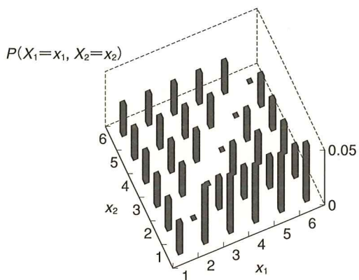
● ——— 図 3.9 2 回目に細工のあるサイコロを振るときの結合確率分布
